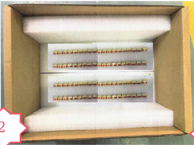
图二，将组件按图示装入箱内。一格 23 个，一层四格，放 4 层，一箱一共 368 个
